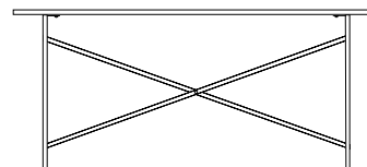
Eiermann 2 Esstisch dining table 1350 x 780 x 720
