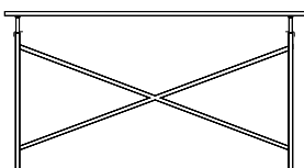
Eiermann 1 1100 x 660/780 x 660 Eiermann 2 1350 x 660/780 x 660
